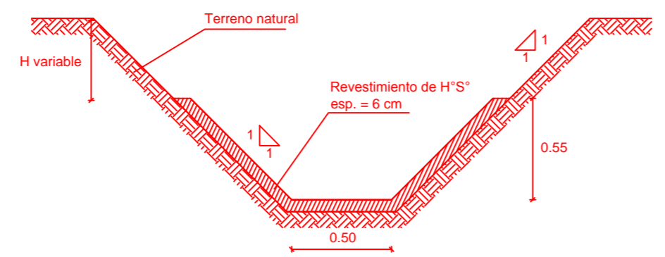
SECCIÓN TIPO 2 (a)
