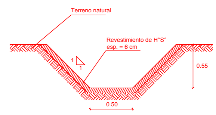
SECCIÓN TIPO 2 (b)
